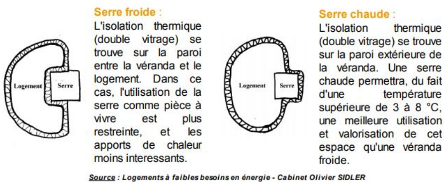
Figure 4 : Schémas explicatifs des différences techniques entre serre froide et serre chaude. Source : Logements à faibles besoins en énergie – Cabinet Olivier SIDLER, 2010.
