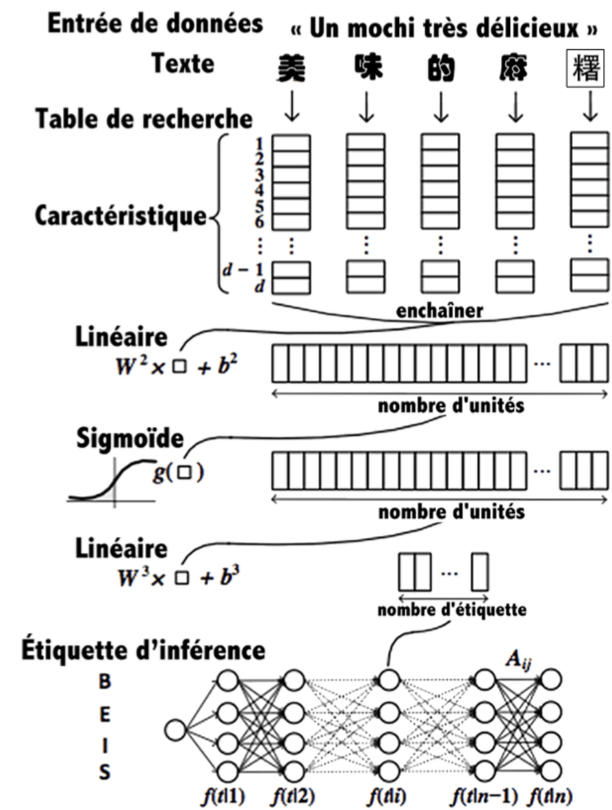
Figure 3 : Procédure de l'analyse des significations scripturaires.
