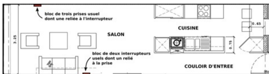
Figure 2 : Situation de l'interrupteur coupeur de prises dans le logement. Source : Renault, 2012.
