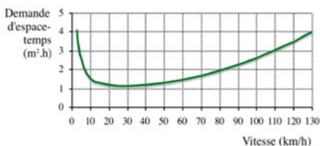
Figure 1 : Consommation d'espace-temps d'une automobile en fonction de sa vitesse. Source : Frédéric Hérin et Emmanuel Ravalet 2008.
