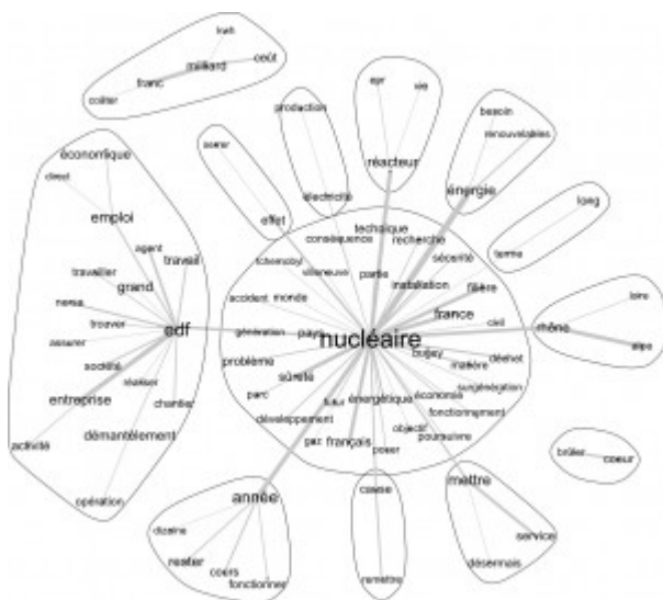
Figure 8 : Analyse de similitude de la classe 2. Source : Romain J. Garcier et
