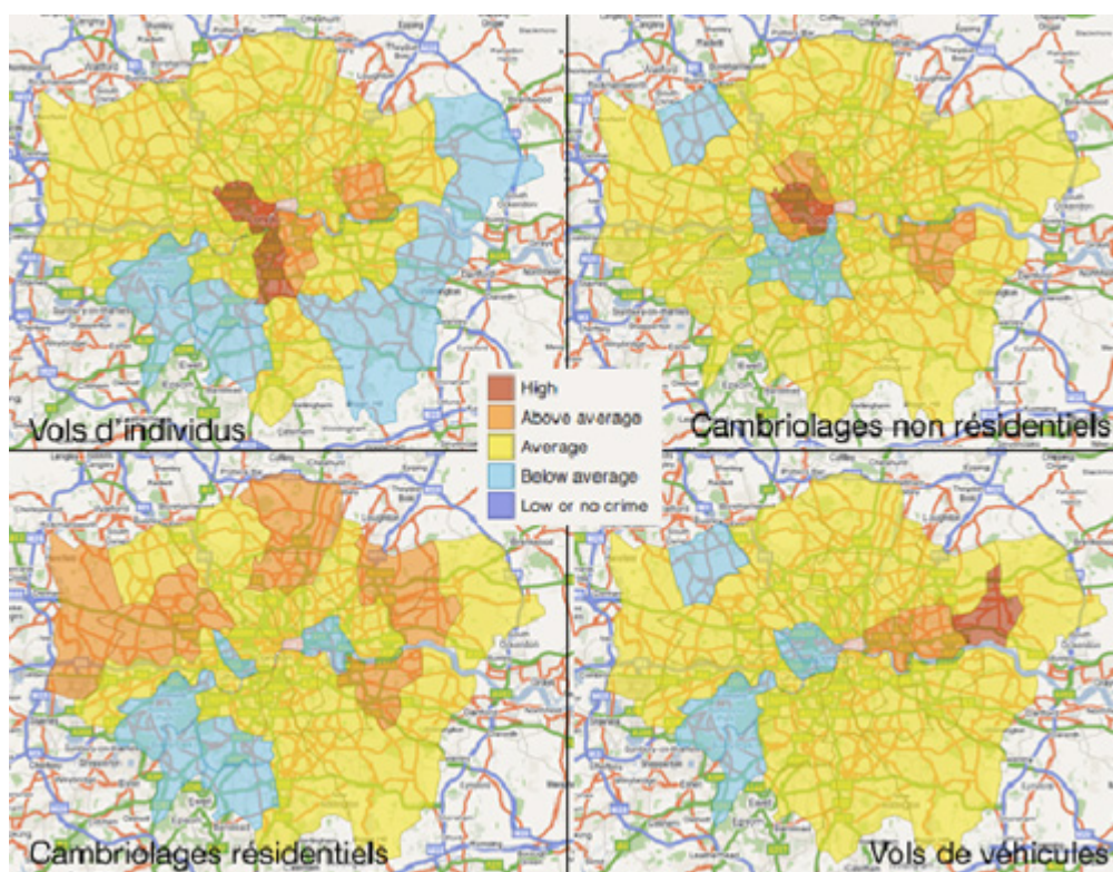
Fig. 4 : London Crime
